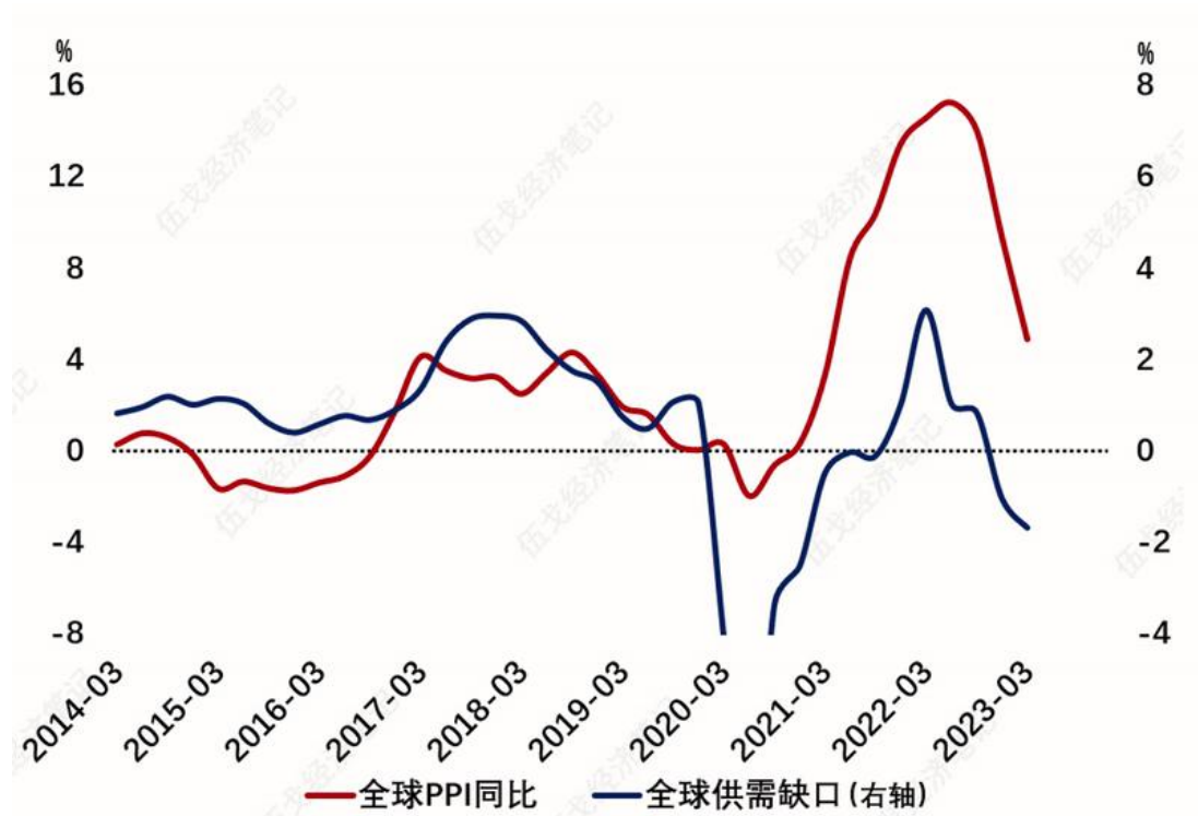
图 2. 全球已现供过于求
